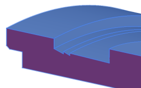
상하고정 하부 케이싱 KEY 상세
